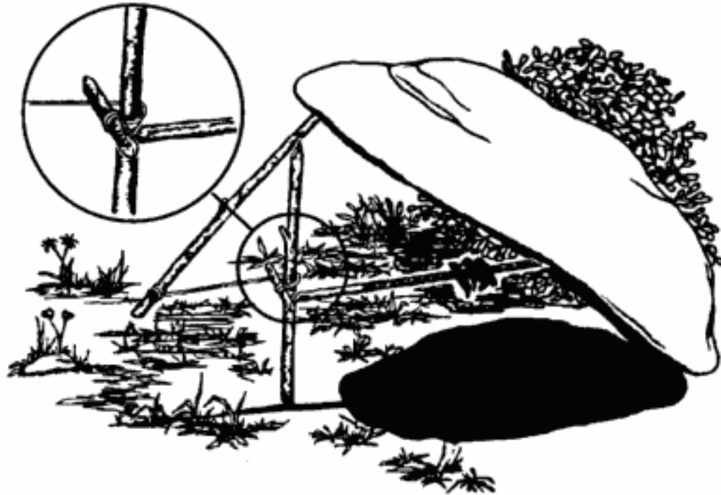
Paiute Dead Fall
