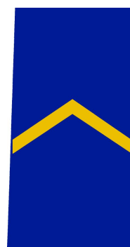
CADET (CDT)
